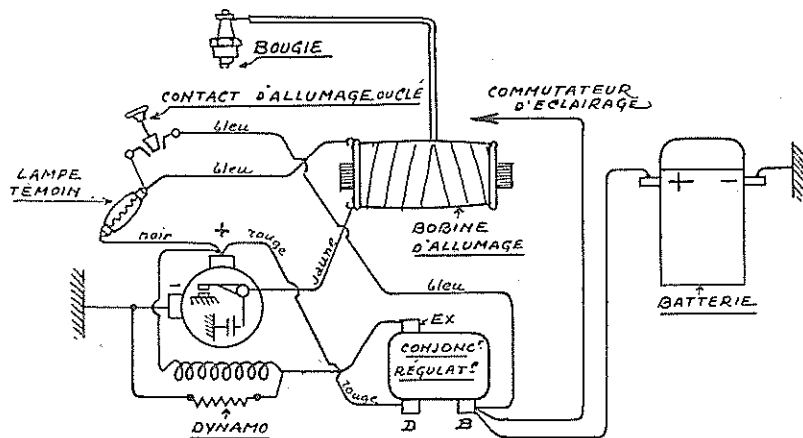
SCHEMA d'ÉQUIPEMENT ELECTRIQUE DYNAMO " MOREL " DV-40
