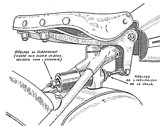
Réglage de la selle sur M 4 T.D. et M 4 T.M.
