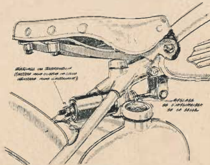
Réglage de la selle sur M3T et M4TD
