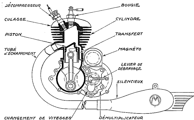
Schéma du moteur 2 vitesses
