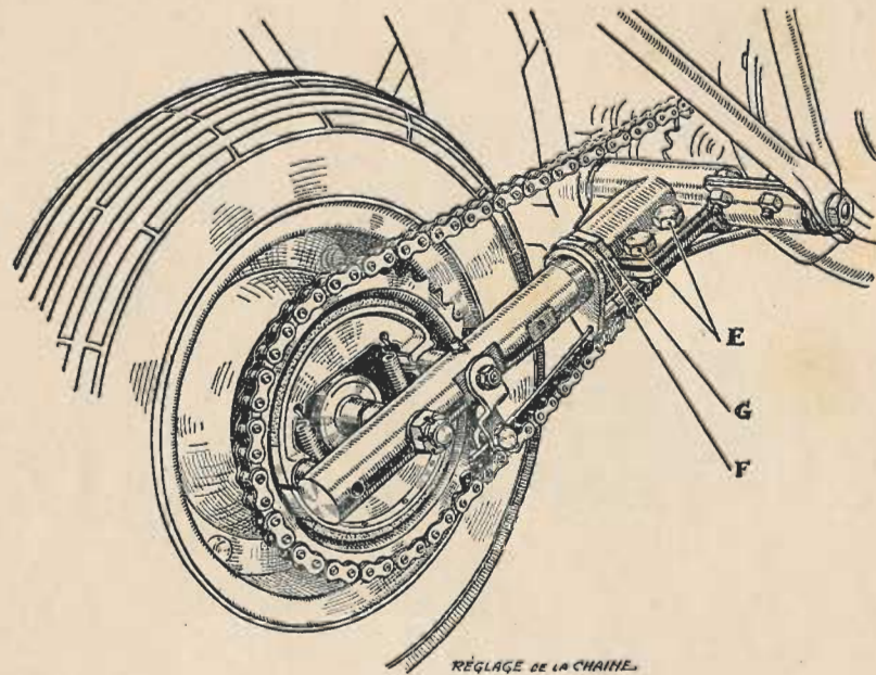
RÉGLAGE DE LA CHAÎNE.
