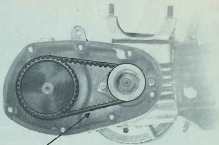
COURROIE DENTELÉE EN CAOUTCHOUC ARMÉ, SOUPLE ET SILENCIEUSE.
